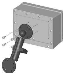
Доп. кронштейн (опция) (возможна поставка P/N 403180)
