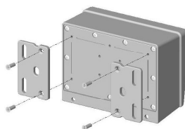
Боковая крепёжная планка (в комплекте)
