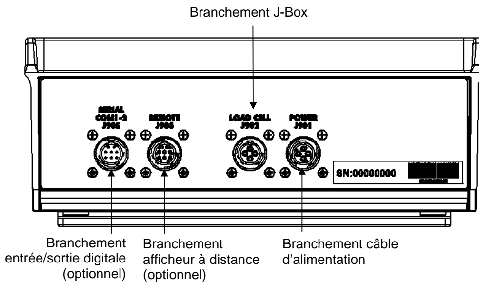
Figure 3 : Branchement de câbles panneau inférieur
