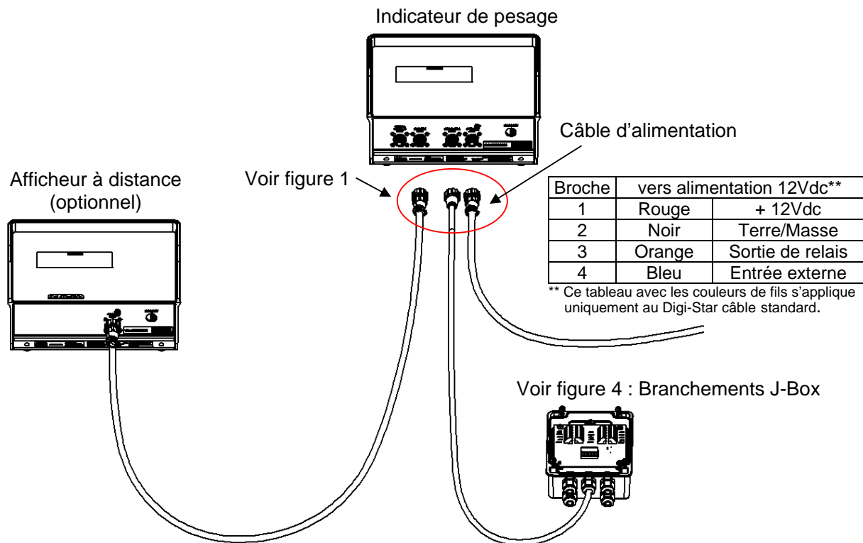
Figure 2 : Schéma de branchement indicateur de pesage
